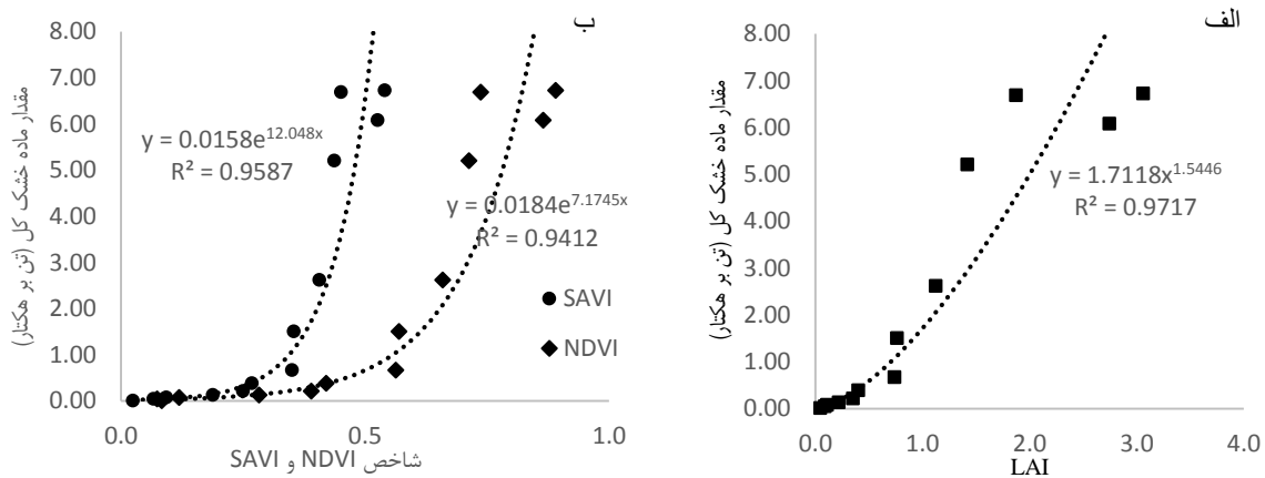
شکل ۵- رابطه بین مقدار ماده خشک اندازه‌گیری شده با LAI (الف) و NDVI و SAVI (ب) برآورد شده از تصاویر ماهواره‌ای سنتینل ۲ طی دوره رشد
